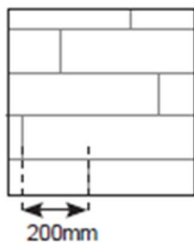
Kuva 3a. Puukuviointi: Lankut tulee asentaa satunnaisesti porrastetuin päätysaumoain, jotka ovat vähintään 200 mm:n päässä toisistaan.
